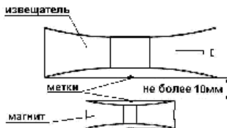
Рис. 7 Общий вид, установочные и присоединительные размеры
