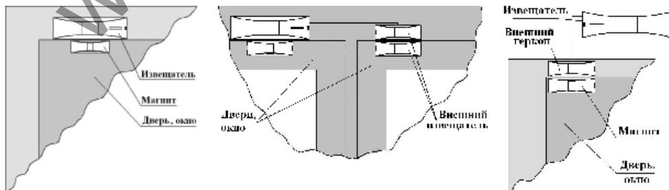
Рис.9 Варианты размещения «Полус-Р2»
