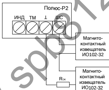
Рис. 8 – Схема подключения
